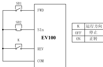
图 6-11 三线式运转模式 1 示意图
