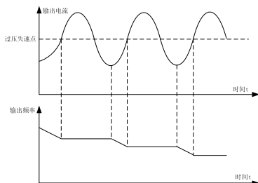
图 6-28 过压失速功能
