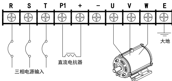
e) 55KW-75KW 变频器主回路端子台配线图 (如图 4-2e)
