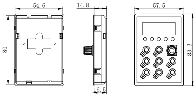
图 1-4 键盘操作器外形及安装尺寸图
