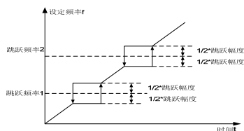
图6-16 跳跃频率示意图
