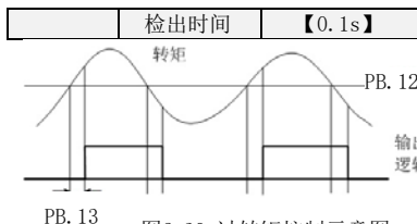
图6-30 过转矩控制示意图
