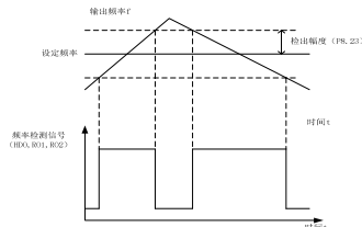
图 6-20 频率到达检出幅度示意图
