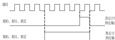
图 6-18 设定计数值和指定计数值示意图
