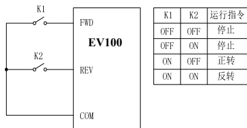
图 6-10 两线式运转模式 2 示意图
