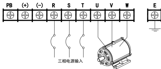
e) 55KW-75KW 变频器主回路端子台配线图 (如图 4-2e)
