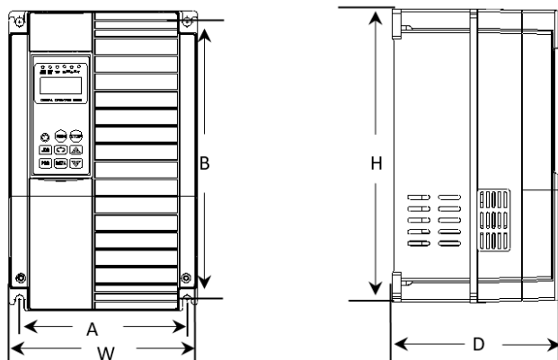
图 1-3 变频器外形尺寸示意图
