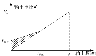
图 6-7 手动转矩提升示意图
