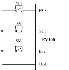
图6-12 三线式运转模式2示意图
