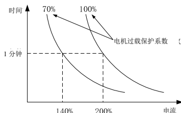
图6-27 电机过载保护系数设定
