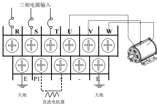
g) 132KW-315KW 变频器主回路端子台配线图 (如图 4-2g)
