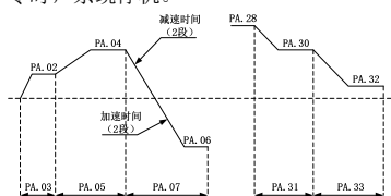
图6-24 简易PLC示意图
