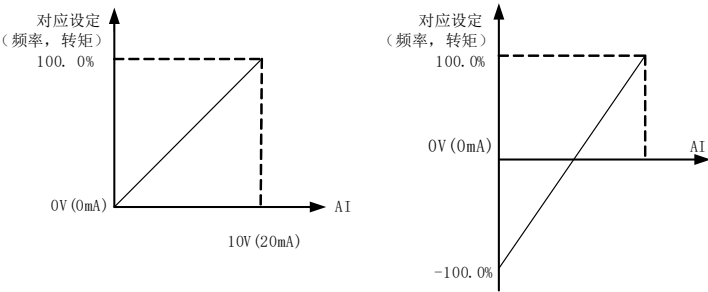
图 6-12 模拟给定与设定量的对应关系
