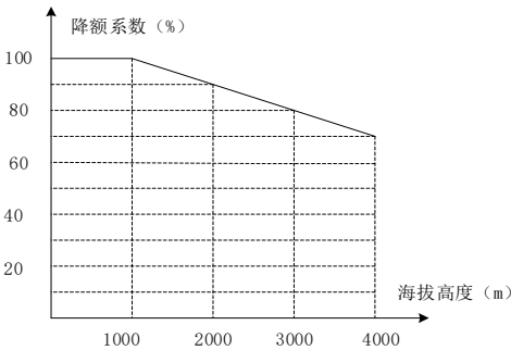
图 1-5 变频器海拔高度降额曲线图
