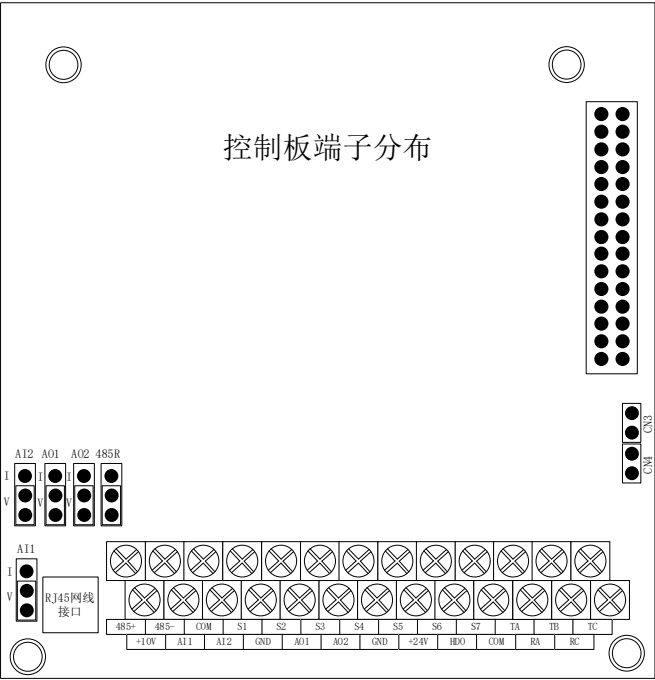
图 3-6 控制端子分布图
