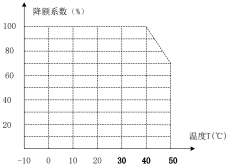
图 1-4 变频器温度降额曲线图
