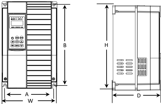
图 2-4 变频器外形尺寸示意图
