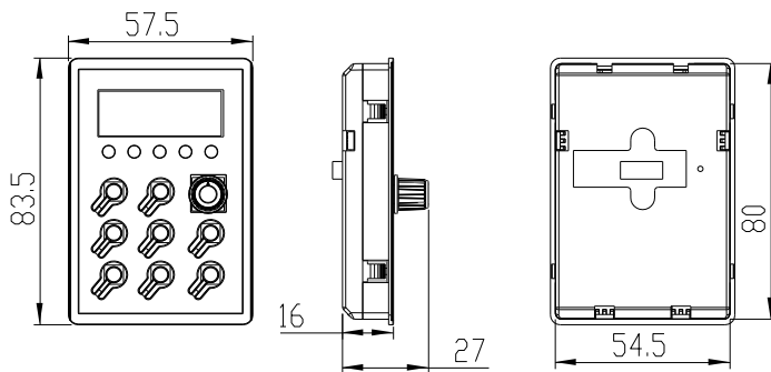
图 2-5 键盘操作器外形及安装尺寸图
