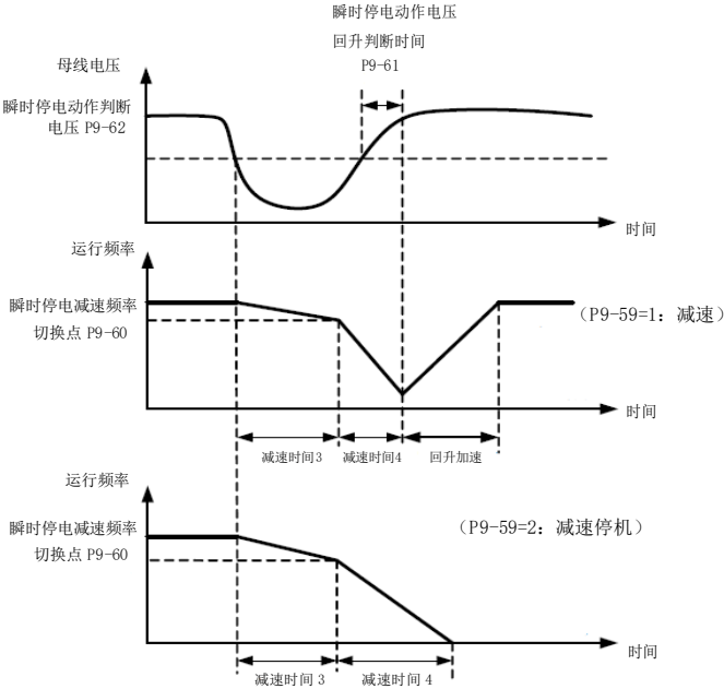
图 6-24 瞬时停电动作示意图
