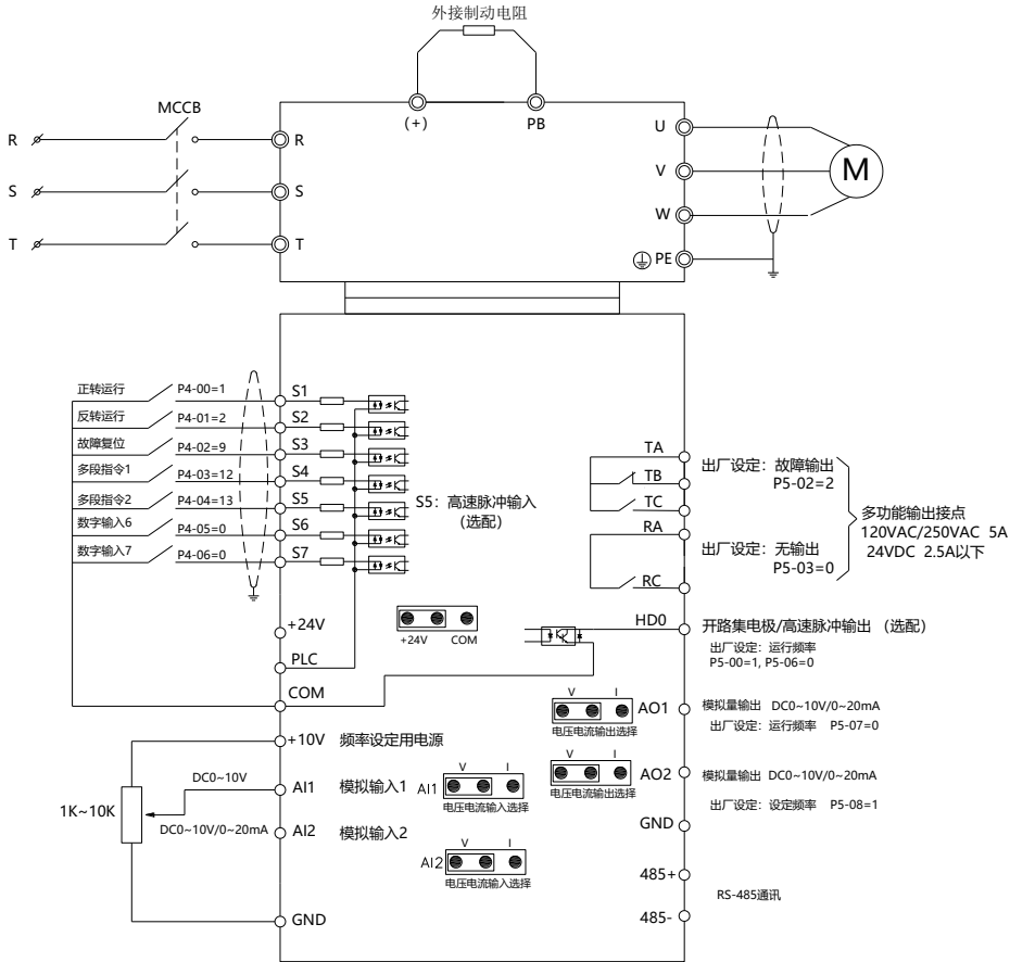
图 3-5 标准接线图
