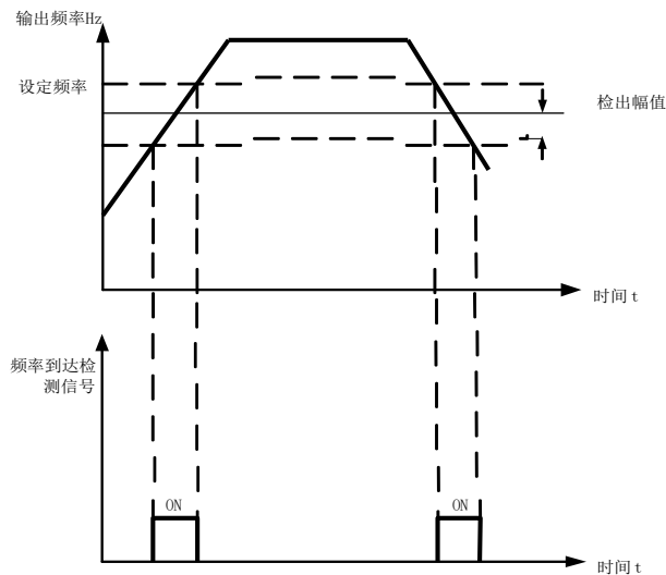
图 6-17 频率到达检出幅值示意图
