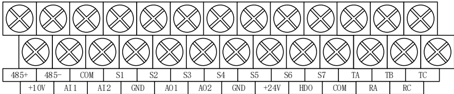
图3-4 控制回路接线端子图
