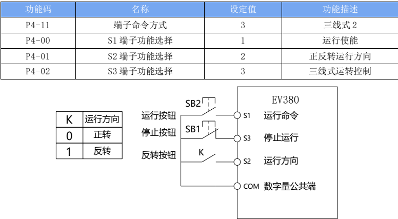
图 6-11 三线式控制模式 2
