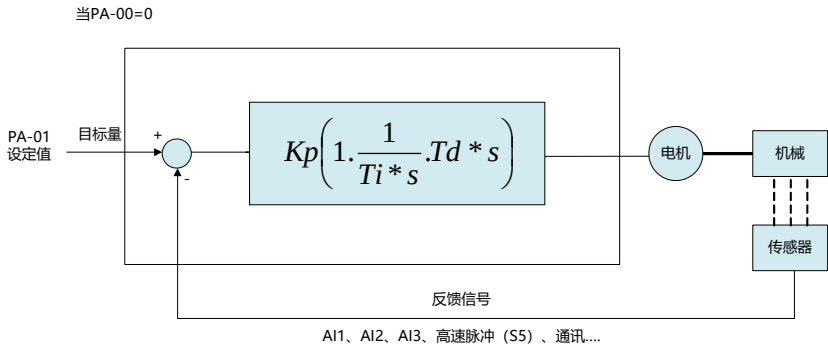
图 6-25 过程 PID 原理框图
