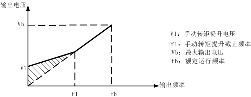
图 6-5 手动转矩提升示意图
