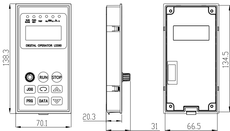
图 2-6 键盘操作器外形及安装尺寸图
