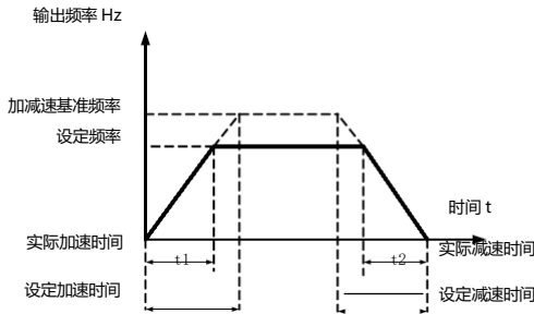
图 6-3 加减速时间示意图
