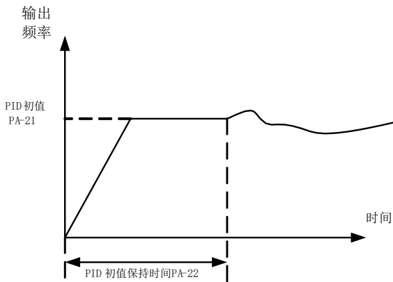
图 6-27 PID 初值的功能示意图
