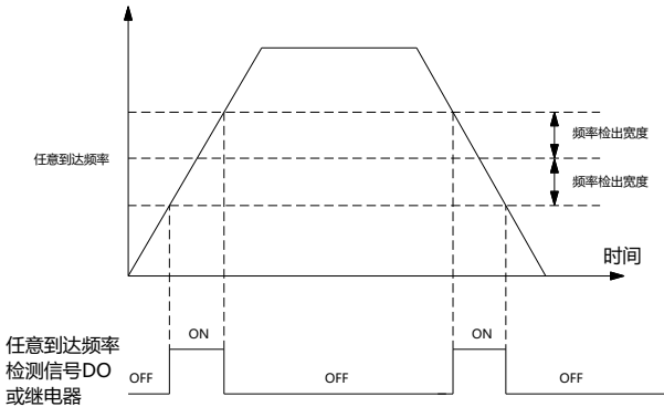
图 6-20 任意到达频率检测示意图
