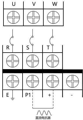
i) 350KW-630KW 变频器主回路端子排配线图（如图 3-3i）
