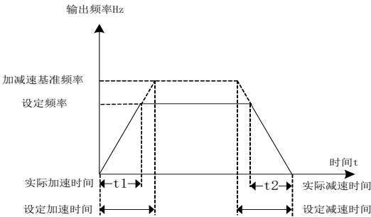
图 6-3 加减速时间示意图
