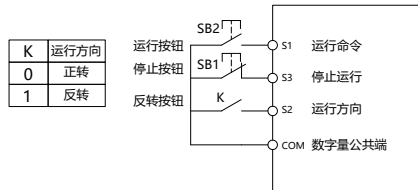
图 6-11 三线式控制模式 2
