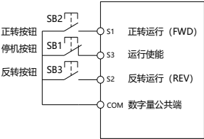
图 6-10 三线式控制模式 1
