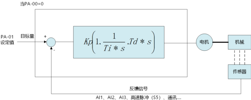
图 6-25 过程 PID 原理框图
