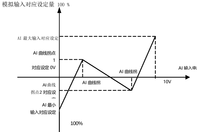
图 6-31 曲线 4 和曲线 5 示意图
