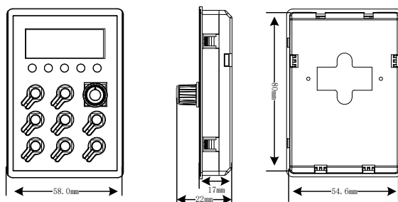
图 2-6 键盘操作器外形及安装尺寸图（11KW 以下）
