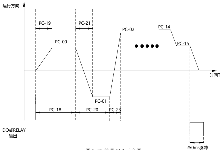
图 6-30 简易 PLC 示意图
