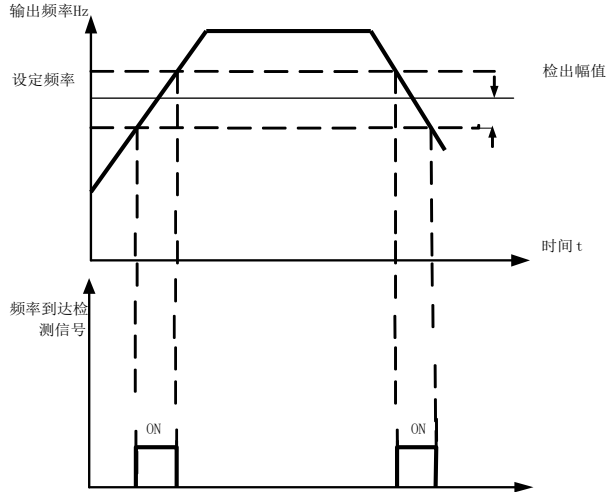
图 6-17 频率到达检出幅值示意图
