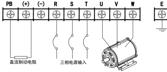
f) 55KW-75KW 变频器主回路端子排配线图 (如图 3-3f)
