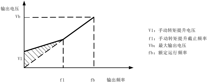
图 6-5 手动转矩提升示意图
