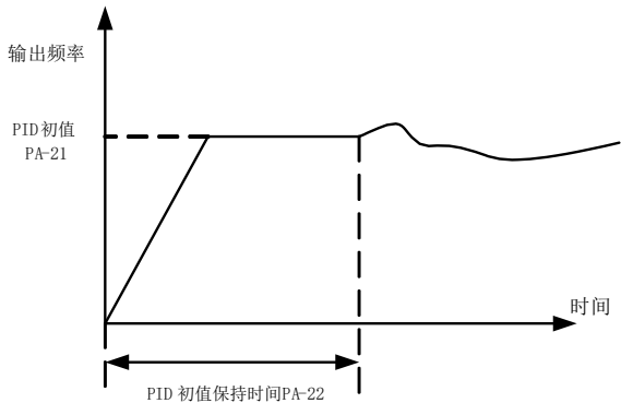
图 6-27 PID 初值的功能示意图
