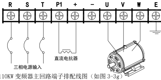
g) 90KW-110KW 变频器主回路端子排配线图 (如图 3-3g)
