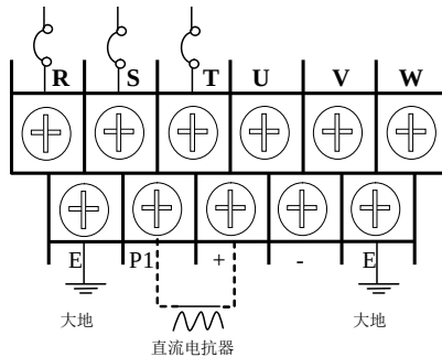
h) 132KW-315KW 变频器主回路端子排配线图 (如图 3-3h)
