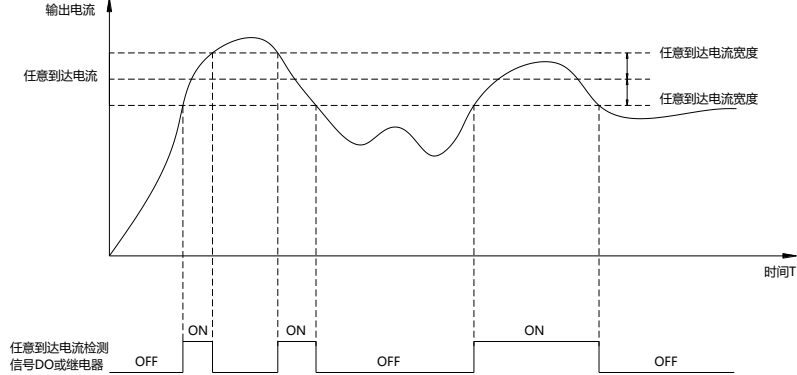
图 6-23 任意到达电流检测示意图
