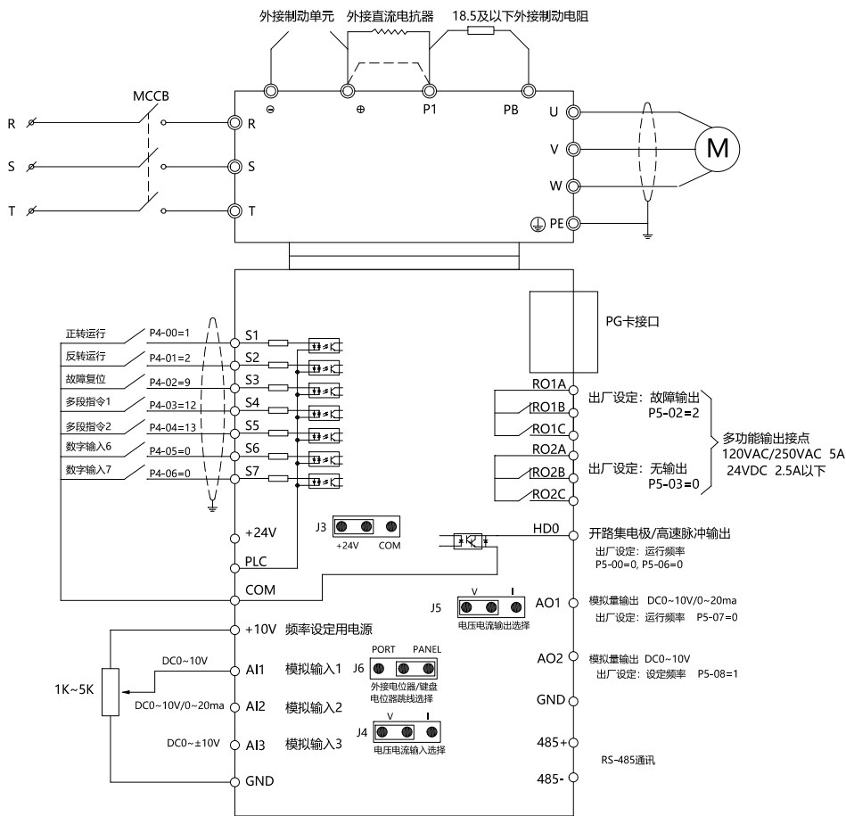
图 3-5 标准接线图
