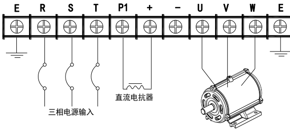
h) 132KW-315KW 变频器主回路端子排配线图 (如图 3-3h)
